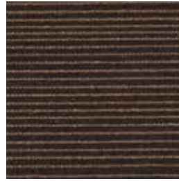
Americano GAN-07
